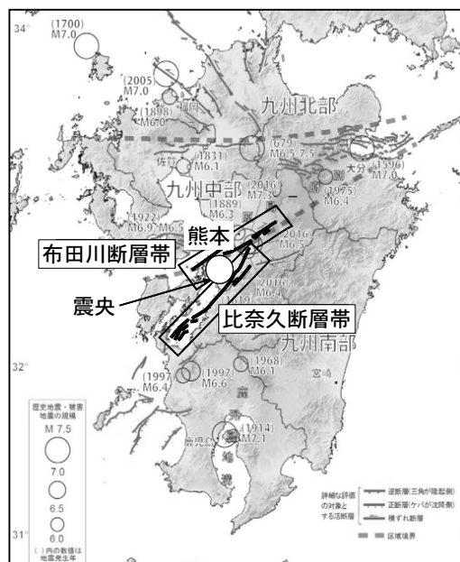
【出典：地震調査研究推進本部 地震調査委員会 (令和8年7月)】
