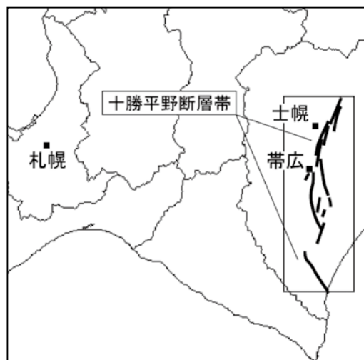
【出典：地震調査研究推進本部 地震調査委員会 (平成17年4月)】
