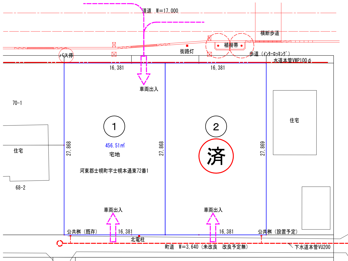
新生 定住促進宅地 区画平面図
